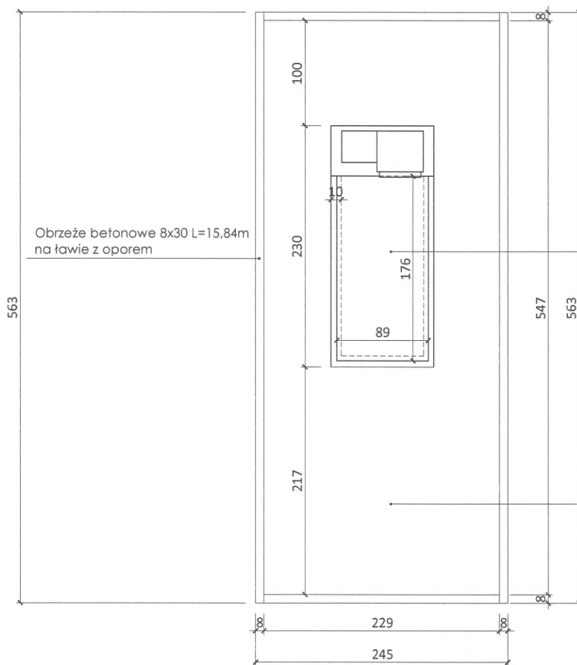
RZUT POZIOMY
