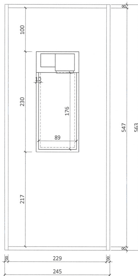
RZUT POZIOMY
